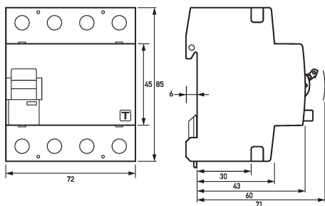
Maßzeichnung Fehlerstromschutzschalter DFS 4 016-4/0,03-B NK HD
