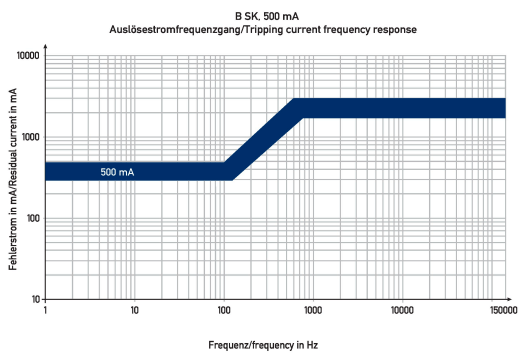
Diagramme Fehlerstromschutzschalter DFS 4 016-4/0,50-B SK
