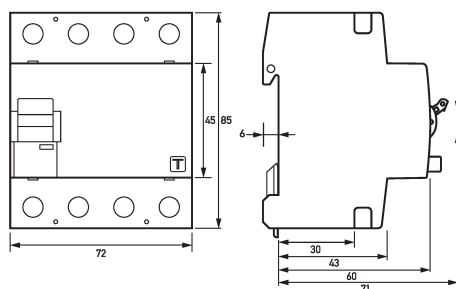
Maßzeichnung Fehlerstromschutzschalter DFS 4 025-4/0,03-A V500
