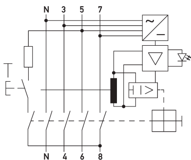
Schaltungsbeispiel Fehlerstromschutzschalter DFS 4 025-4/0,03-B SK
