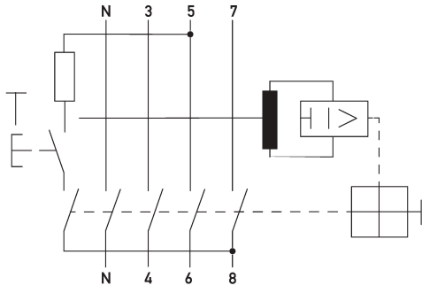
Schaltungsbeispiel Fehlerstromschutzschalter DFS 4 025-4/0,10-A V500
