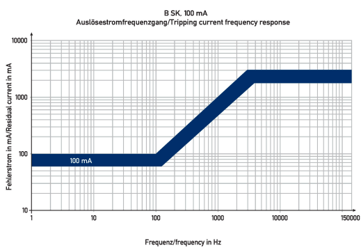
Kennlinie B SK 100 mA
