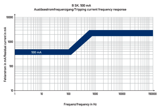
Diagramme Fehlerstromschutzschalter DFS 4 025-4/0,50-B SK V500
