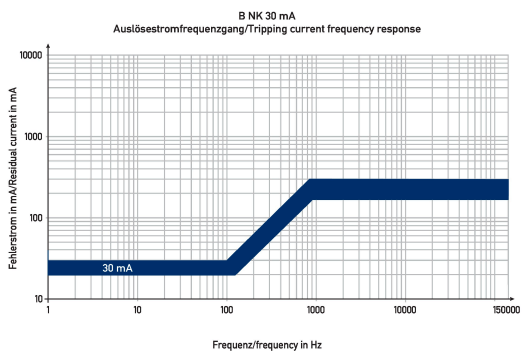
Diagramme Fehlerstromschutzschalter DFS 4 040-4/0,03-B NK HD
