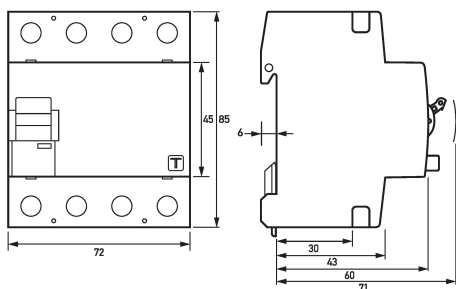
Maßzeichnung Fehlerstromschutzschalter DFS 4 040-4/0,03-B NK V500
