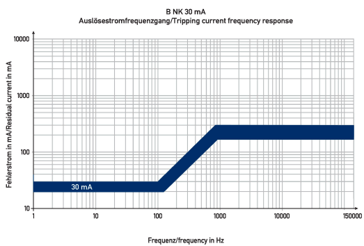
Diagramme Fehlerstromschutzschalter DFS 4 040-4/0,03-B NK V500
