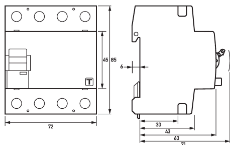
Maßzeichnung Fehlerstromschutzschalter DFS 4 040-4/0,03-B SK
