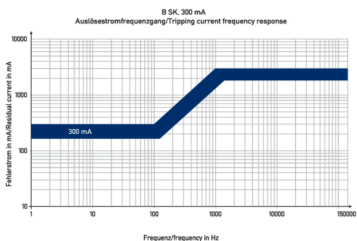
Diagramme Fehlerstromschutzschalter DFS 4 040-4/0,30-B SK S V500
