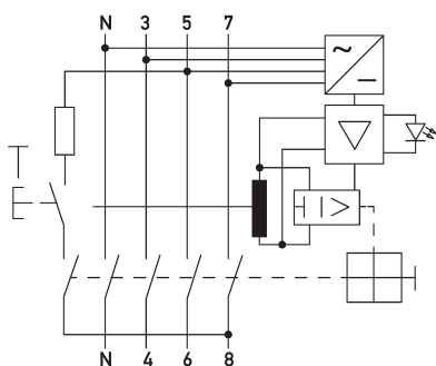
Schaltungsbeispiel Fehlerstromschutzschalter DFS 4 040-4/0,30-B SK S V500
