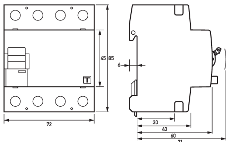
Maßzeichnung Fehlerstromschutzschalter DFS 4 040-4/0,30-B SK S V500
