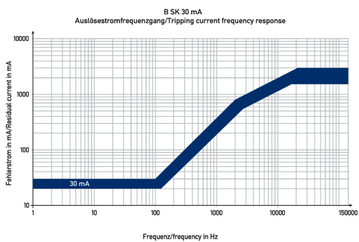
Diagramme Fehlerstromschutzschalter DFS 4 063-4/0,03-B SK HD
