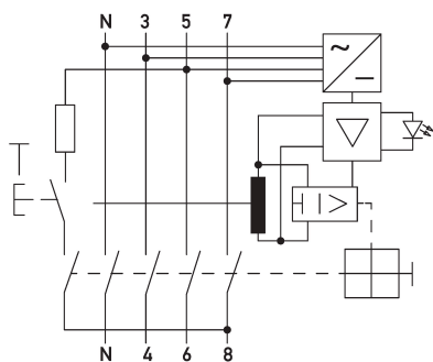
Schaltungsbeispiel Fehlerstromschutzschalter DFS 4 063-4/0,30-B SK V500
