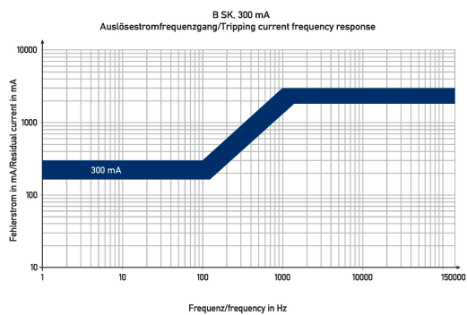
Diagramme Fehlerstromschutzschalter DFS 4 063-4/0,30-B SK V500
