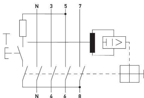
Schaltungsbeispiel Fehlerstromschutzschalter DFS 4 063-4/0,50-A KV
