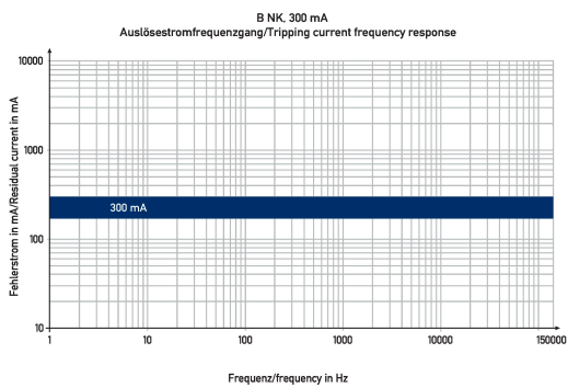
Diagramme Fehlerstromschutzschalter DFS 4 080-4/0,30-B NK V500
