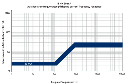
Diagramme Fehlerstromschutzschalter DFS 4 100-4/0,03-B NK
