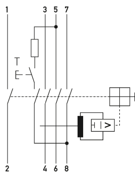
Schaltungsbeispiel Fehlerstromschutzschalter DFS 4W 040-3/0,50-A
