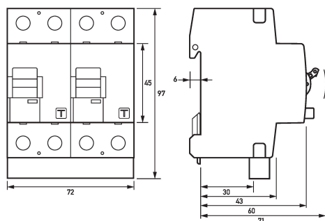
Maßzeichnung Fehlerstromschutzschalter DFS 2 016-2/0,03-A Twin
