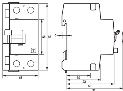
Maßzeichnung Fehlerstromschutzschalter DFS 2 025-2/0,01-A FT
