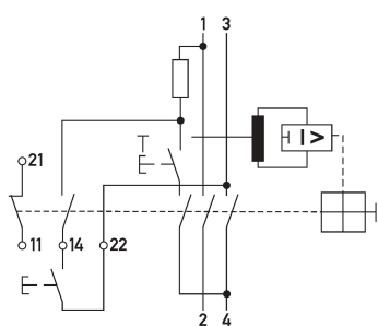
Schaltungsbeispiel Fehlerstromschutzschalter DFS 2 025-2/0,01-A FT
