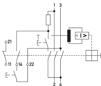
Schaltungsbeispiel Fehlerstromschutzschalter DFS 2 040-2/0,01-A FT
