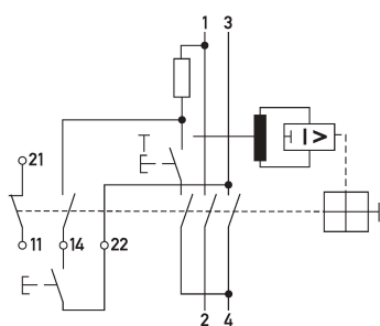
Anschlusschema
