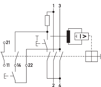
Schaltungsbeispiel Fehlerstromschutzschalter DFS 2 063-2/0,50-A FT
