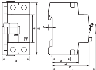
Maßzeichnung Fehlerstromschutzschalter DFS 2 063-2/0,50-A FT
