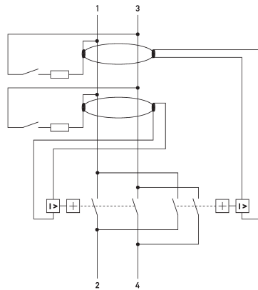
Anschlusschema
