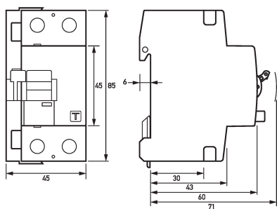
Maßzeichnung Fehlerstromschutzschalter DFS 2 100-2/0,10-A FT
