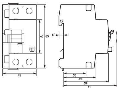
Maßzeichnung Gruppenansicht
