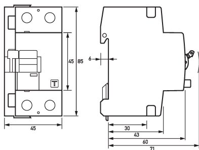
Maßzeichnung Fehlerstromschutzschalter DFS 2 125-2/0,50-A FT
