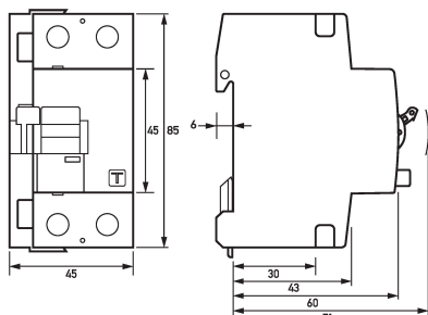
Maßzeichnung Fehlerstromschutzschalter DFS 2 125-2/0,50-A FT
