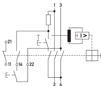
Schaltungsbeispiel Fehlerstromschutzschalter DFS 2 125-2/0,50-A FT
