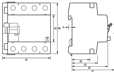
Maßzeichnung Fehlerstromschutzschalter DFS 4 025-4/0,30-A FT
