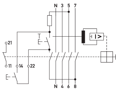
Schaltungsbeispiel Fehlerstromschutzschalter DFS 4 025-4/0,30-A FT
