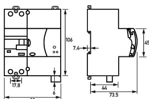
Maßzeichnung Fehlerstromschutzschalter DRCCB 5 ST 025-2/0,03-A
