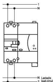
Schaltungsbeispiel Fehlerstromschutzschalter DRCCB 5 ST 025-2/0,03-A
