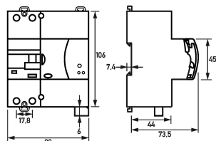
Maßzeichnung Gruppenansicht
