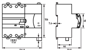
Maßzeichnung Fehlerstromschutzschalter DRCCB 5 STR 040-4/0,03-A
