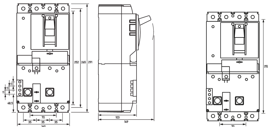
Maßzeichnung Leistungsschalter mit Fehlerstromschutz DFL 8 100-4/0,03-A
