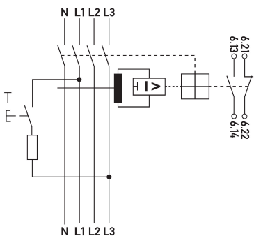
Schaltungsbeispiel Leistungsschalter mit Fehlerstromschutz DFL 8 100-4/0,03-A
