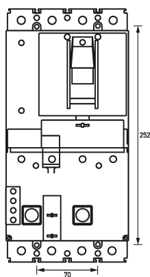
Maßzeichnung Bohrschablone
