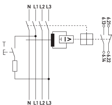
Schaltungsbeispiel Leistungsschalter mit Fehlerstromschutz DFL 8 125-4/0,03-A
