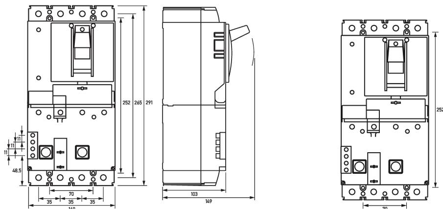
Maßzeichnung Leistungsschalter mit Fehlerstromschutz DFL 8 125-4/0,03-A
