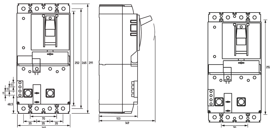
Maßzeichnung Leistungsschalter mit Fehlerstromschutz DFL 8 125-4/X-B NK
