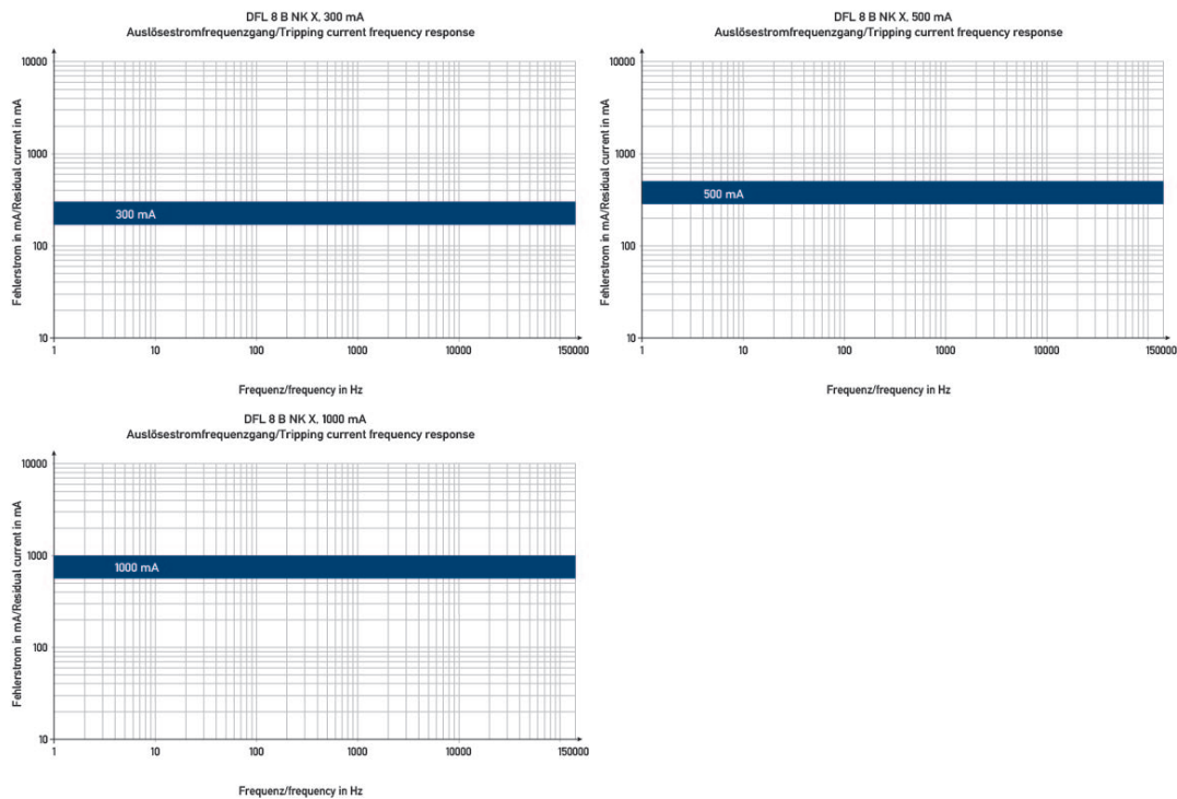
Diagramme Leistungsschalter mit Fehlerstromschutz DFL 8 125-4/X-B NK
