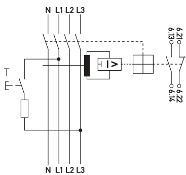
Anschlusschema
