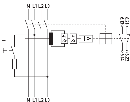
Schaltungsbeispiel Leistungsschalter mit Fehlerstromschutz DFL 8 250-4/X-A
