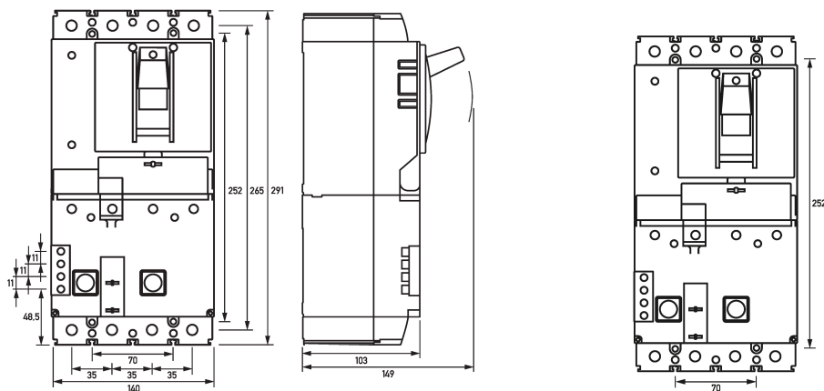
Mazeichnung Leistungsschalter mit Fehlerstromschutz DFL 8 250-4/X-B SK
