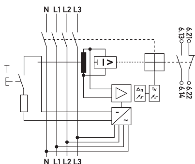
Schaltungsbeispiel Leistungsschalter mit Fehlerstromschutz DFL 8 250-4/X-B SK
