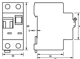
Maßzeichnung FI-/LS-Kombinationen DRCBO 3 Bo6/0,03/1N-A
