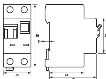
Maßzeichnung Gruppenansicht
