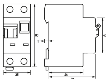
Maßzeichnung FI-/LS-Kombinationen DRCBO 3 B25/0,03/1N-A KV
