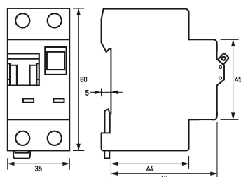
Maßzeichnung FI-/LS-Kombinationen DRCBO 3 B40/0,03/1N-F
