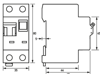
Maßzeichnung FI-/LS-Kombinationen DRCBO 3 C25/0,03/1N-A KV
