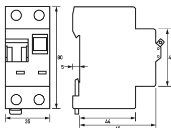
Maßzeichnung FI-/LS-Kombinationen DRCBO 3 C25/0,03/1N-F
