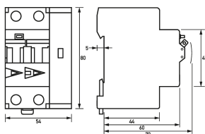
Maßzeichnung Fehlerlichtbogen-Schutzeinrichtungen DAFDD 1 B13/0,03/2-A
