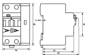
Maßzeichnung Fehlerlichtbogen-Schutzeinrichtungen DAFDD 1 B20/0,03/2-A KV
