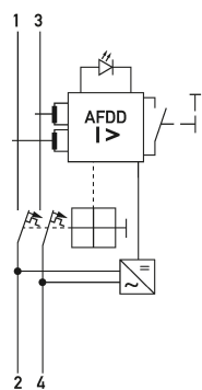
Schaltungsbeispiel Fehlerlichtbogen-Schutzeinrichtungen DAFDD 1 B20/0,03/2-A KV
