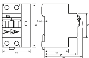
Maßzeichnung Fehlerlichtbogen-Schutzeinrichtungen DAFDD 1 B40/0,03/2-A KV
