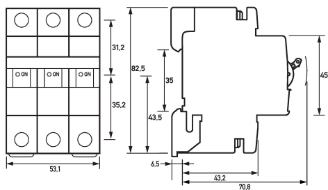
Maßzeichnung Leitungsschutzschalter DLS 6h B13-3
