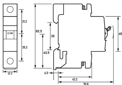
Maßzeichnung Leitungsschutzschalter DLS 6h B16-1
