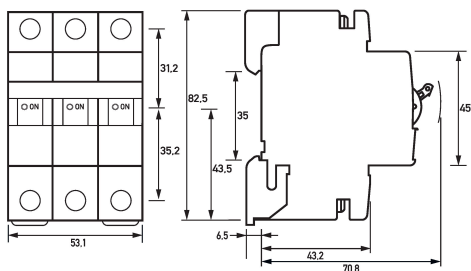
Maßzeichnung Leitungsschutzschalter DLS 6h B16-3
