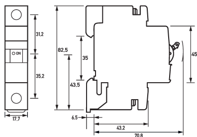
Maßzeichnung Leitungsschutzschalter DLS 6h B25-1
