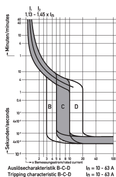
Diagramme Leitungsschutzschalter DLS 6h B25-1
