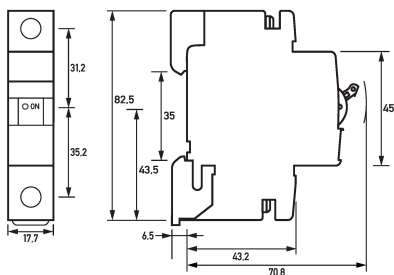
Maßzeichnung Leitungsschutzschalter DLS 6h Bo6-1
