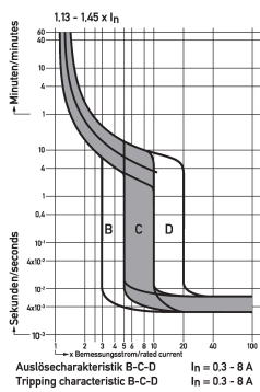
Diagramme Leitungsschutzschalter DLS 6h Bo6-1
